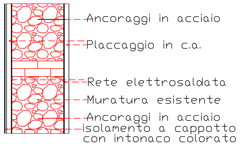
SEZIONE TIPO
